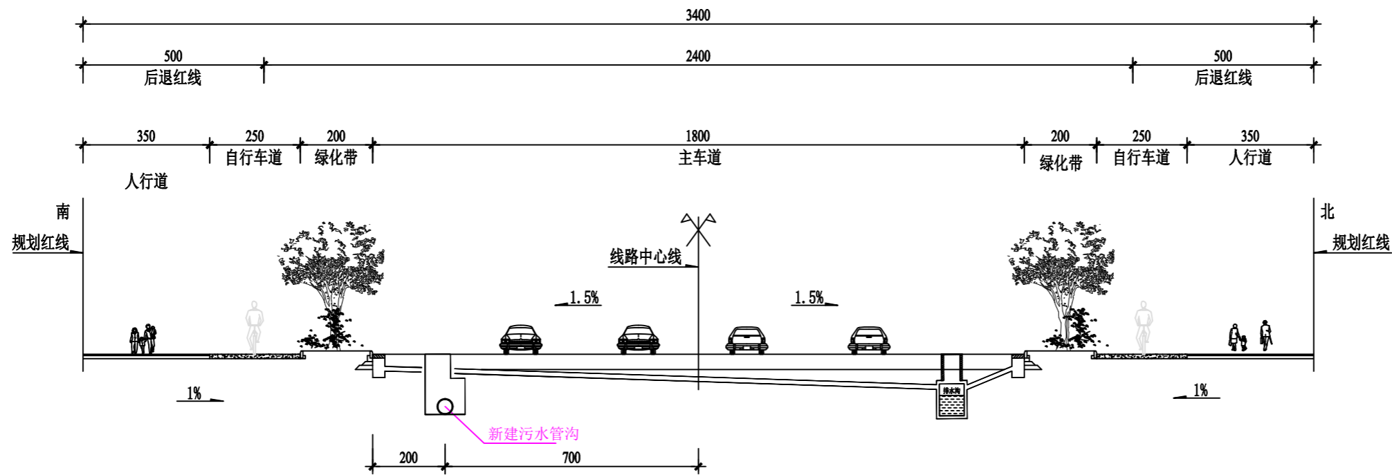
乐善路排水标准横断面示意图
