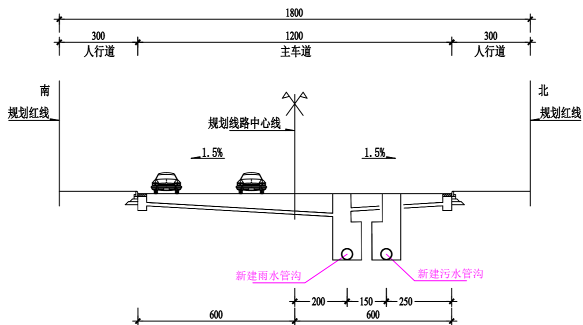
正兴路至客都小学规划路排水标准横断面示意图
