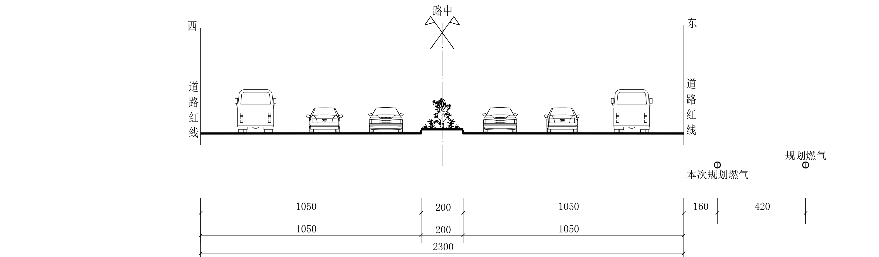
1-1管线综合位置横断面图 (现状道路路幅 单位:cm)
