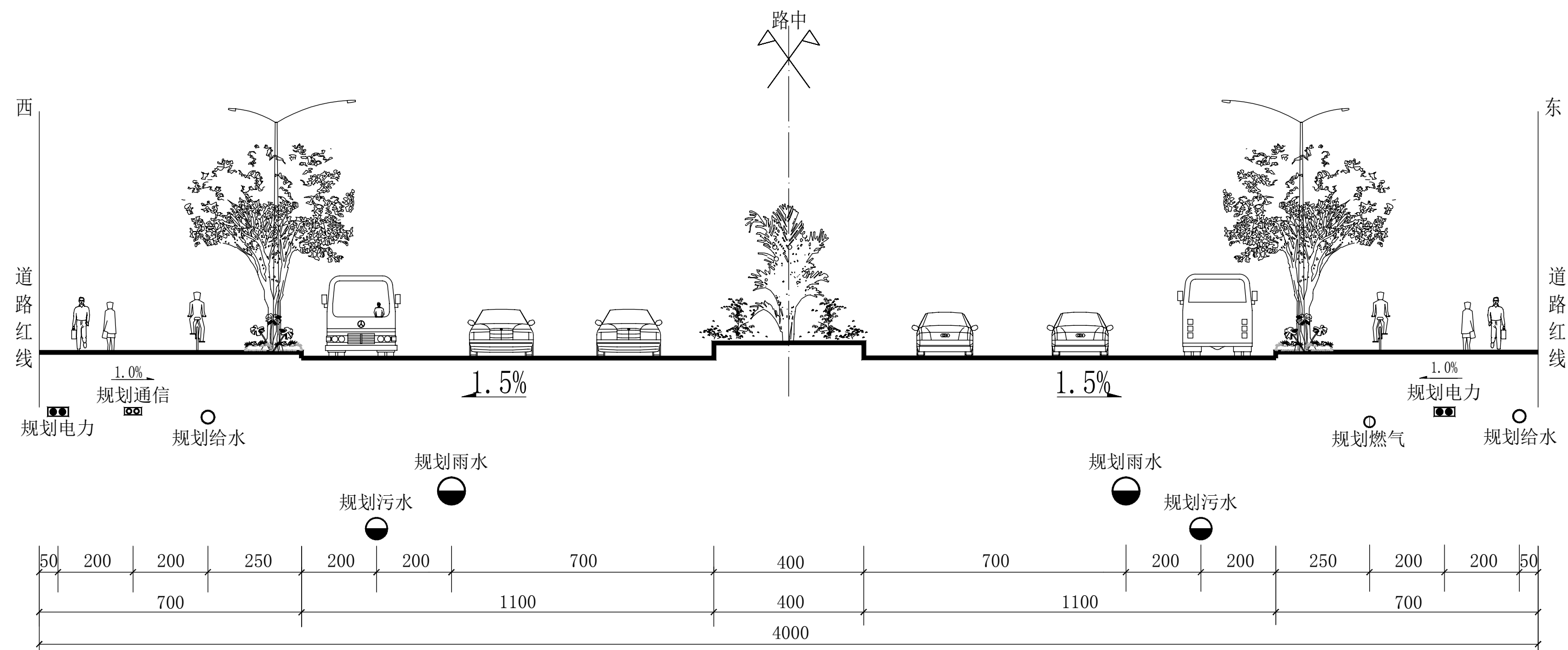
40米道路管线综合位置横断面图 (规划道路路幅 单位:cm)
