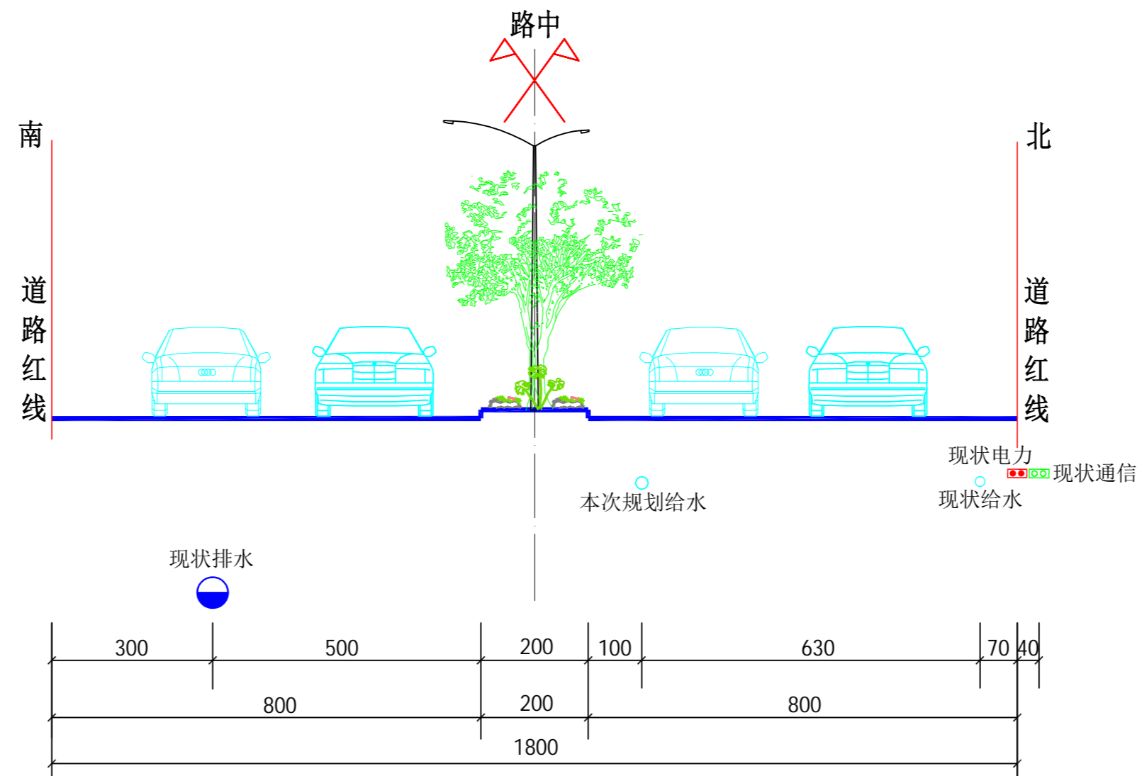
1-1 管线综合位置横断面图 (现状道路路幅 单位: cm)
