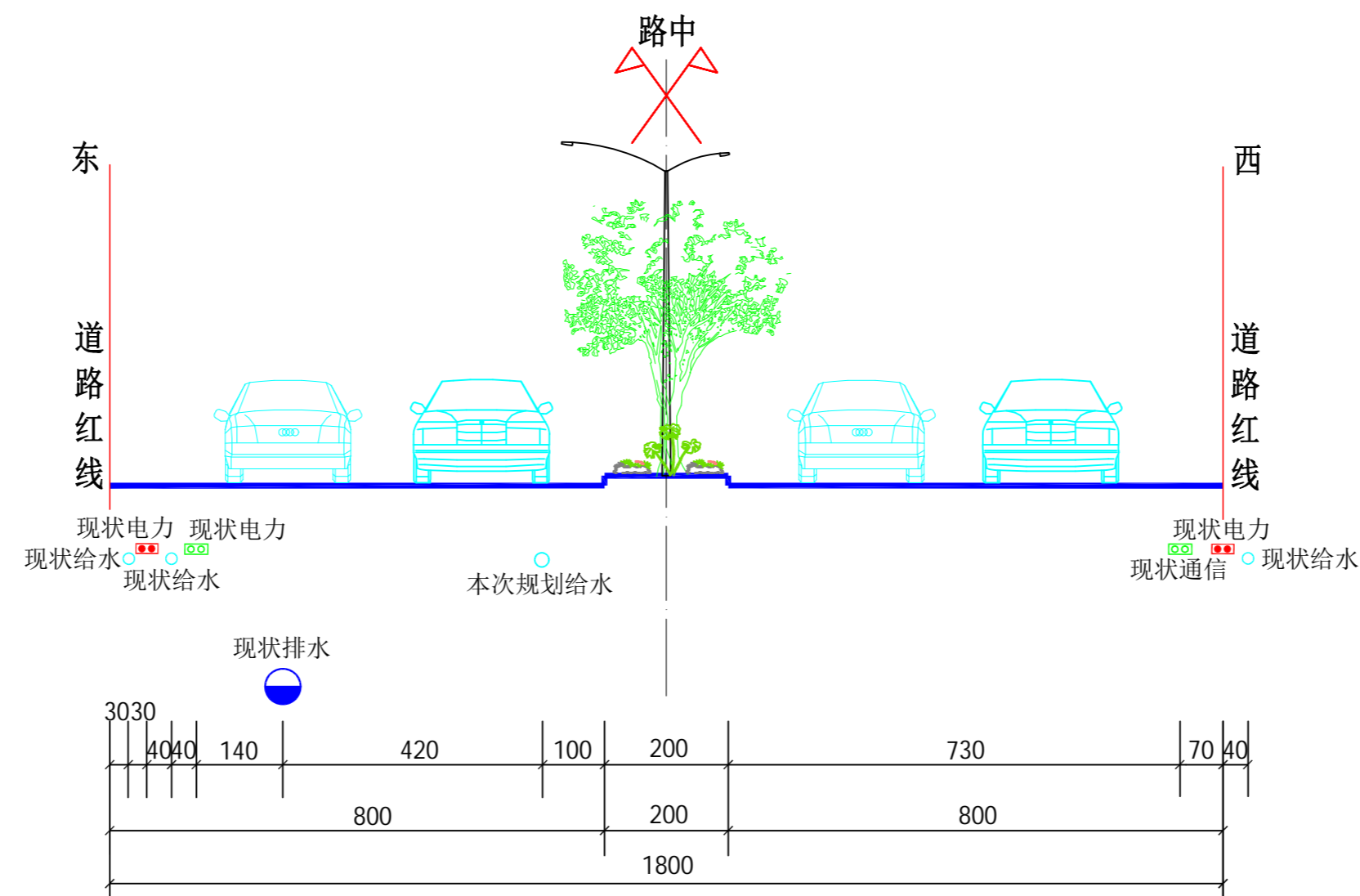
2-2 管线综合位置横断面图 (现状道路路幅 单位: cm)
