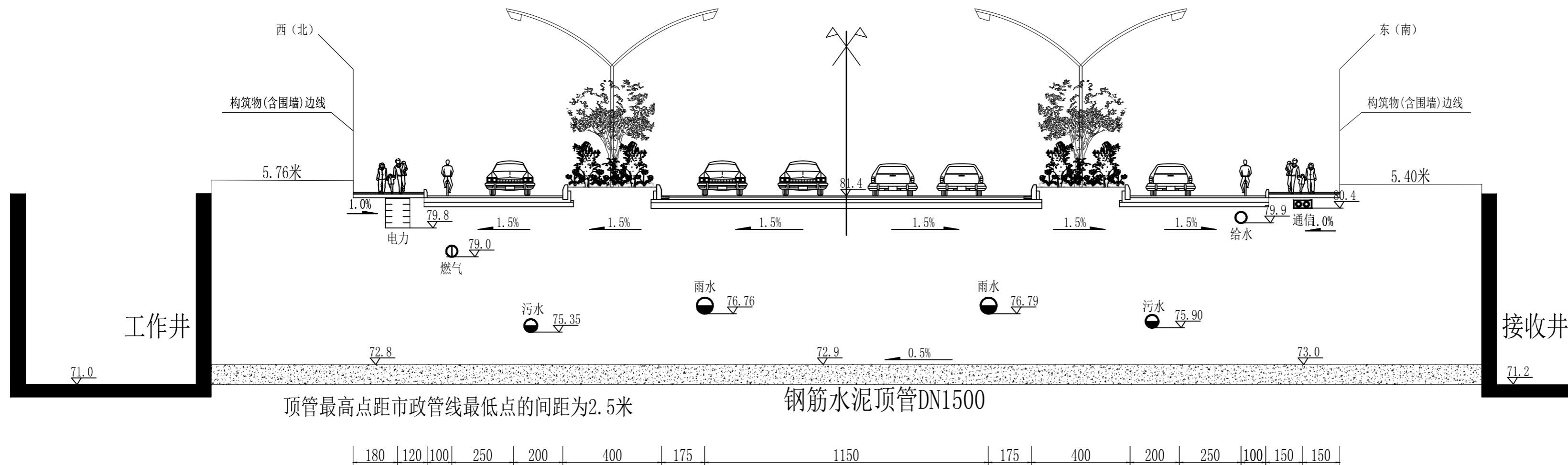
黄塘河西侧新峰路横断面 本图采用长度单位: CM
