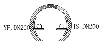
给排水舱
