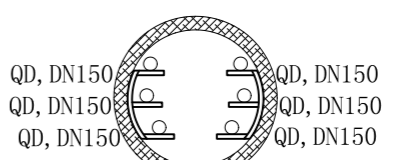
强电舱
