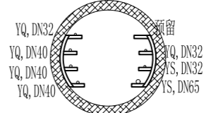
动力舱
