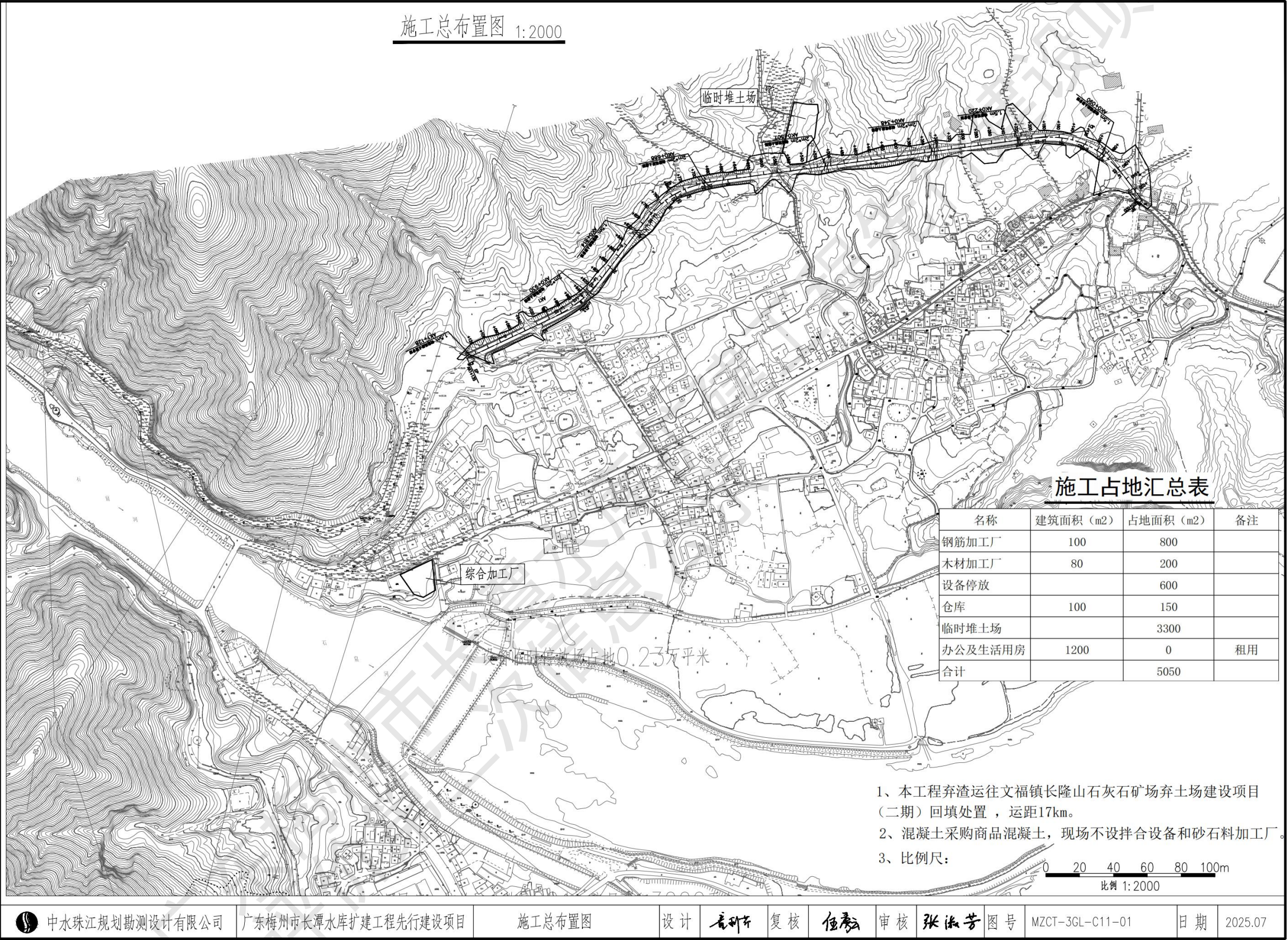
图 3.1-3 施工总布置图
