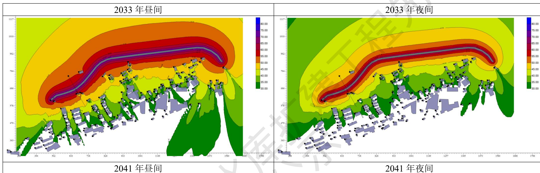
图 5.2-5 项目路段水平等声级线示意图
