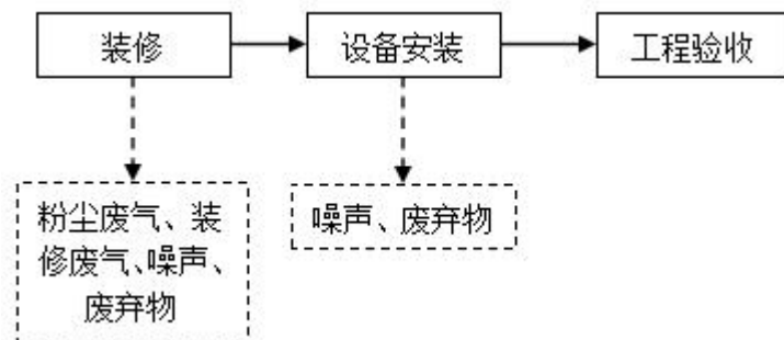
图 2-3 施工期工艺流程图
