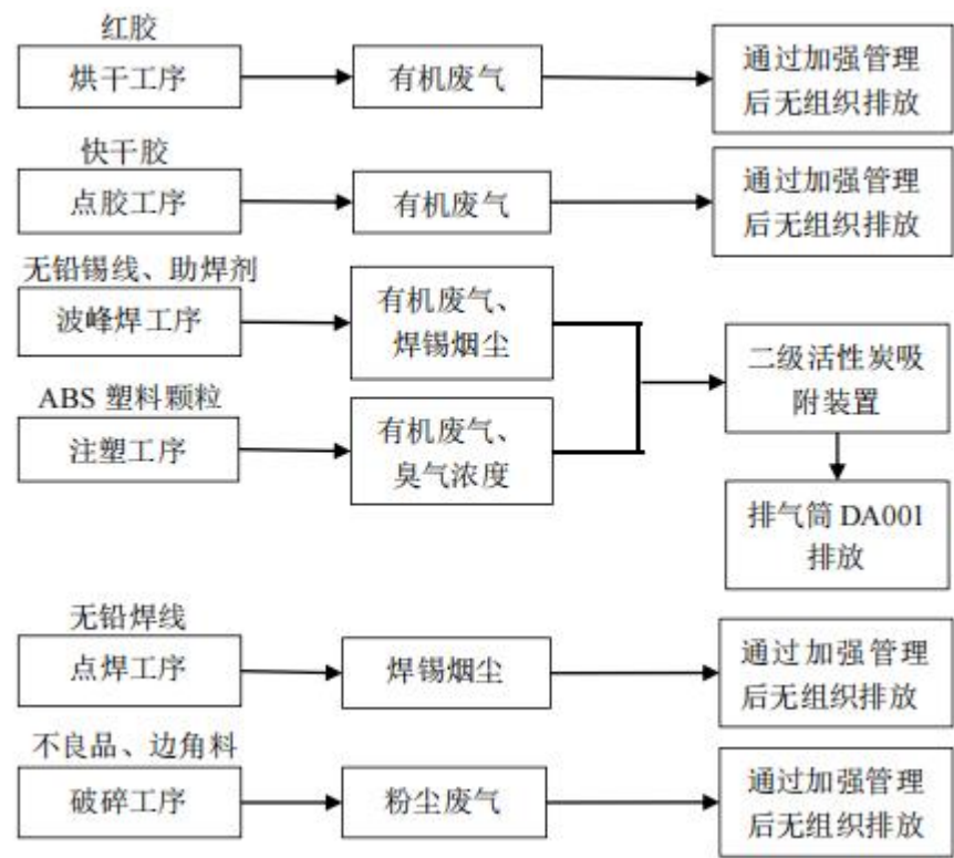
图 4-1 废气处理工艺流程图
