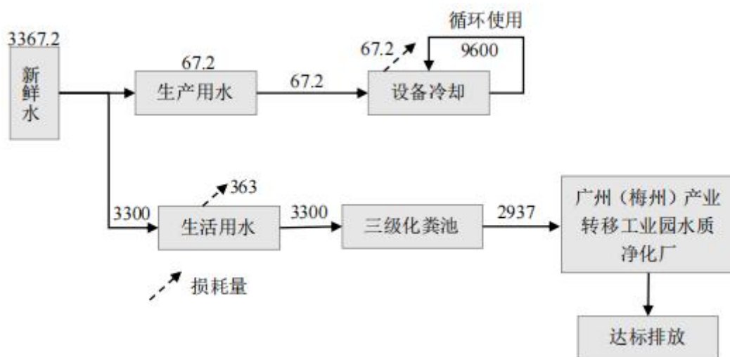
图 2-1 本项目水平衡示意图 单位：m 3 /a
