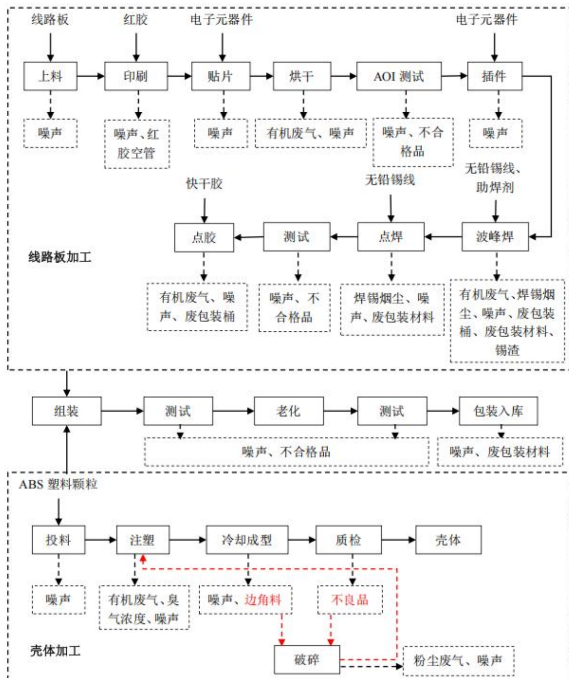
图 2-4 生产工艺与产排污环节图
