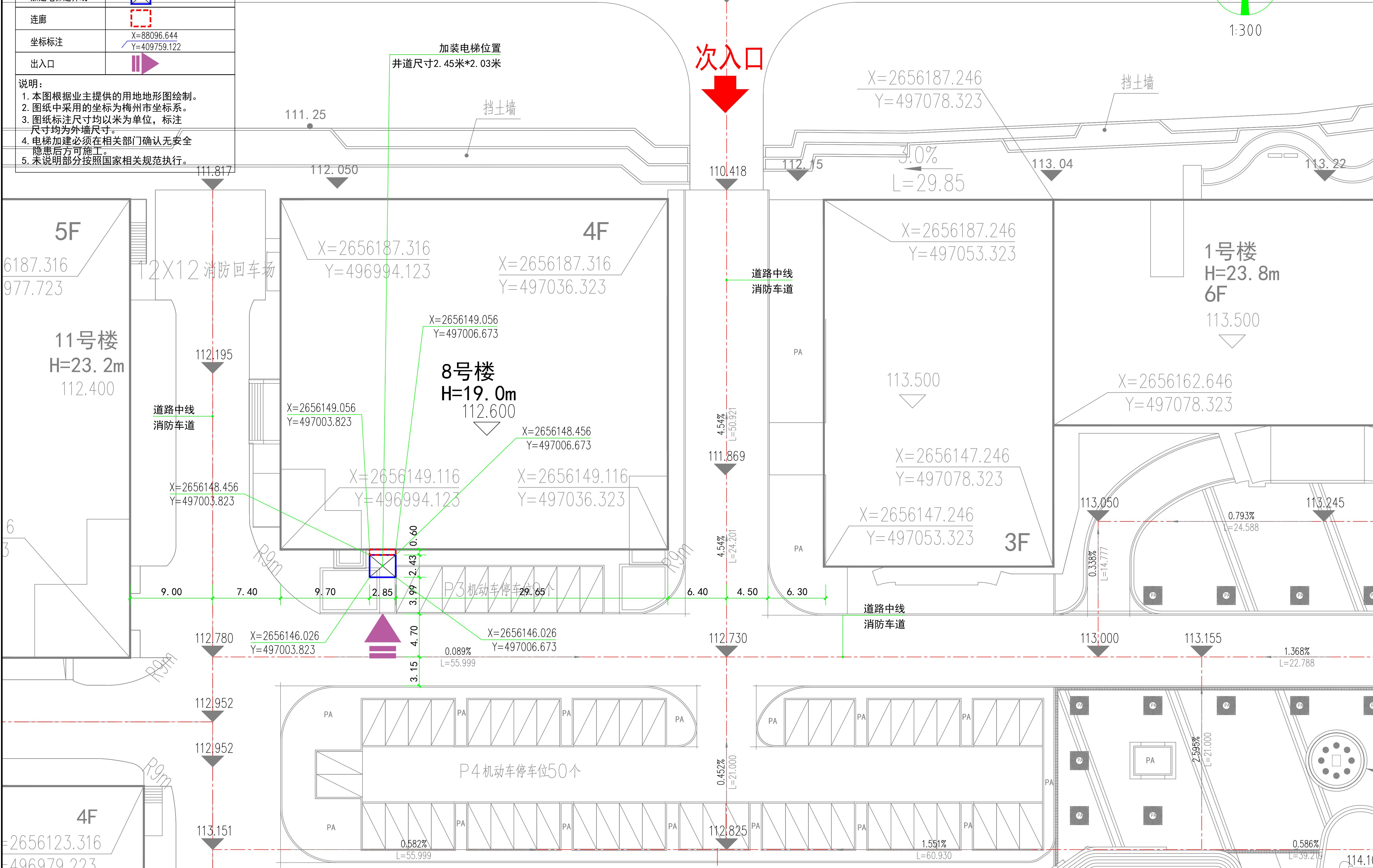
加装电梯位置总平面图 1:300
