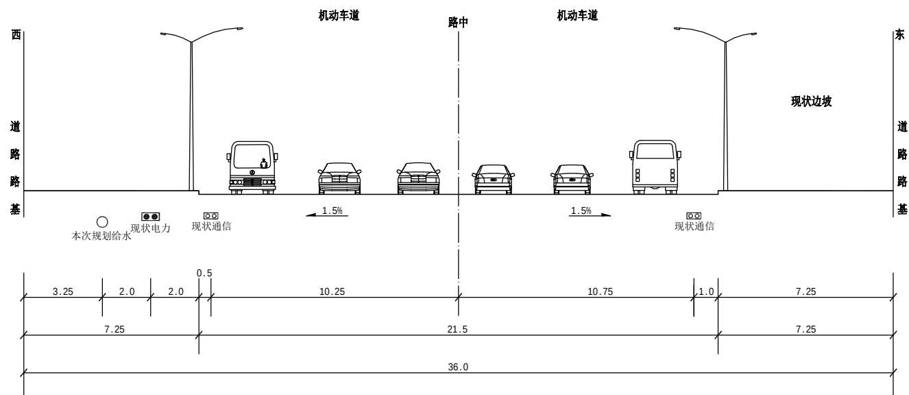
3-3道路管线综合位置横断面示意图
