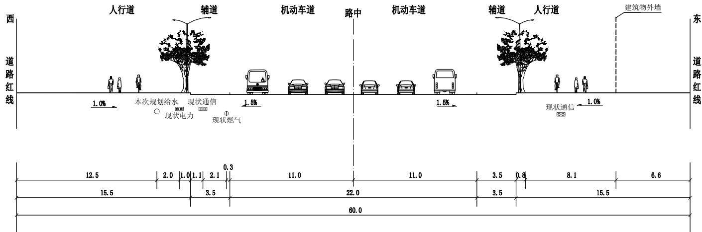
2-2道路管线综合位置横断面示意图 (K1+040 现状 单位:m)
