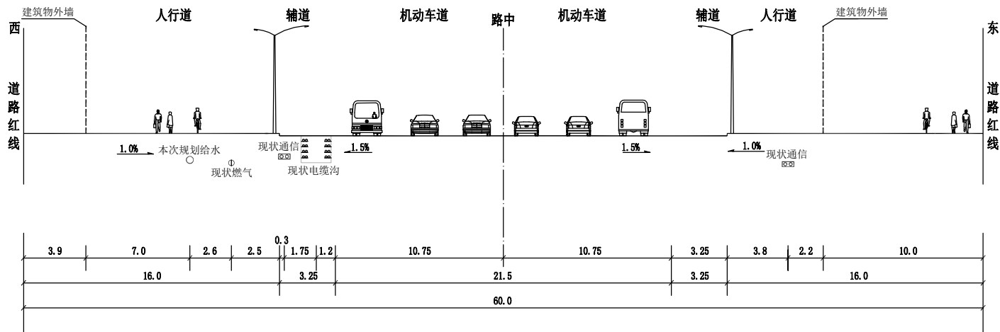
1-1道路管线综合位置横断面示意图 (K0+350 现状 单位:m)
