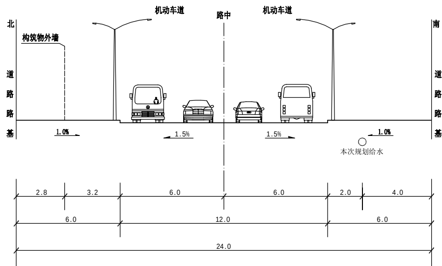
4-4道路管线综合位置横断面示意图
