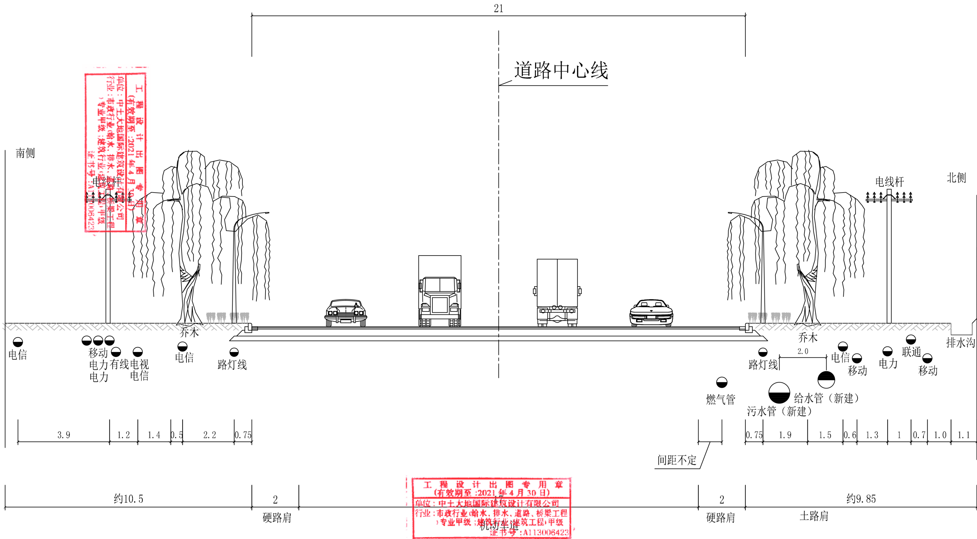
横断面示意图（梅县拘留所门前）
